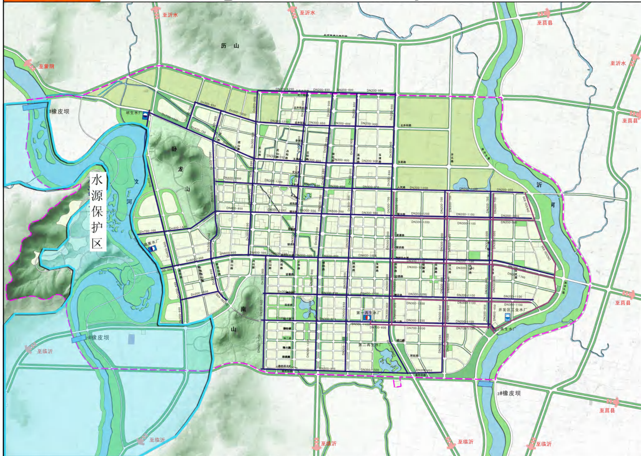
中心城给水规划图
