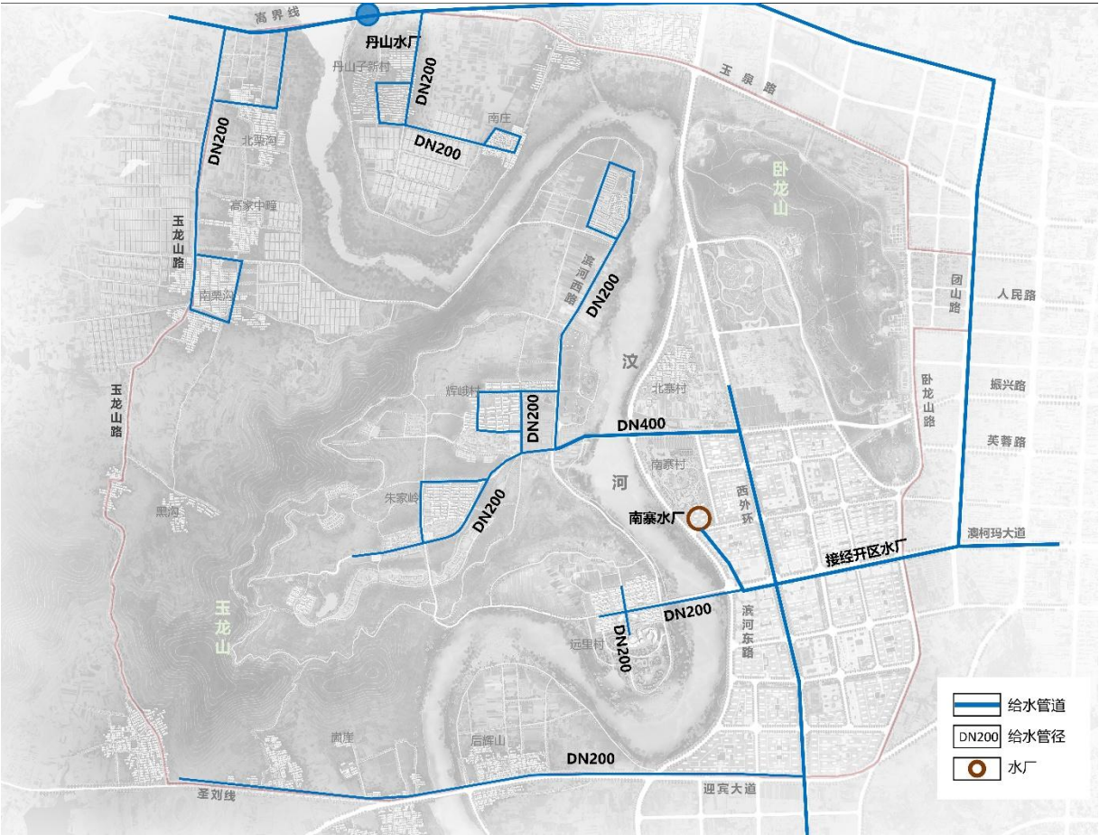
图 6-20 供水工程规划
