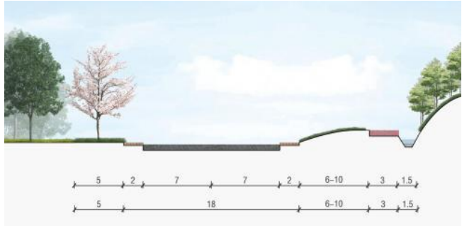
图 6-6 卧龙山西侧环线标准断面
