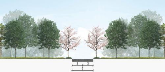
图 6-4 景区二级路标准断面
