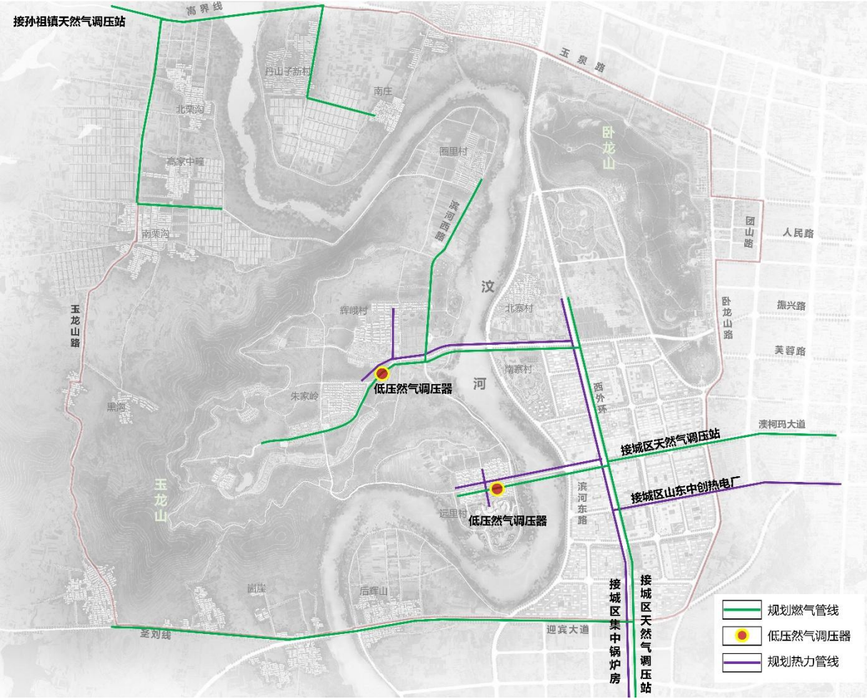
图 6-24 热力燃气设施规划图
