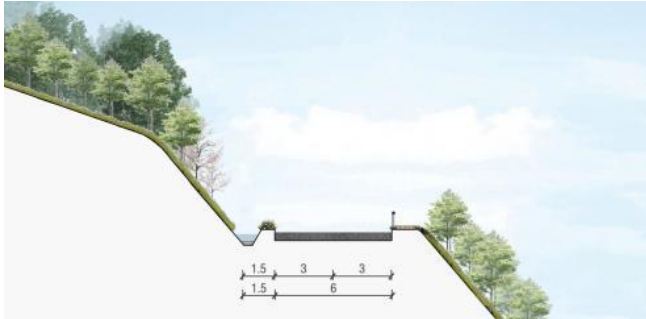
图 6-5 玉龙山环山路标准断面
