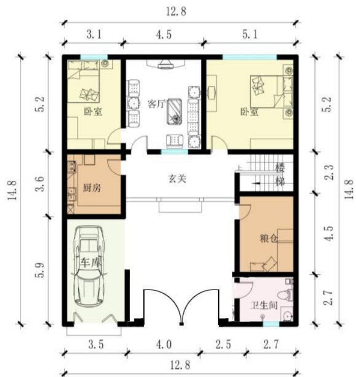
一层平面图
