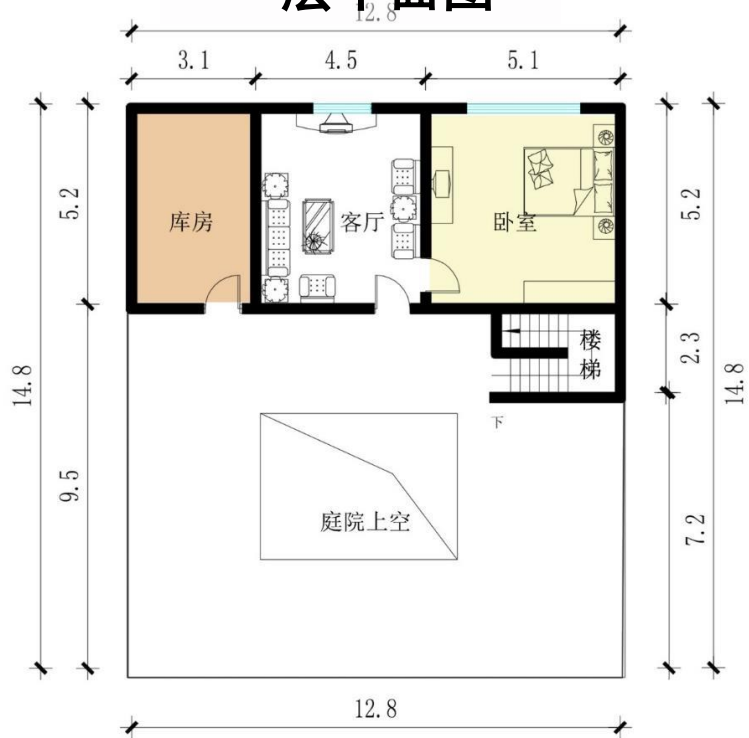
二层平面图
